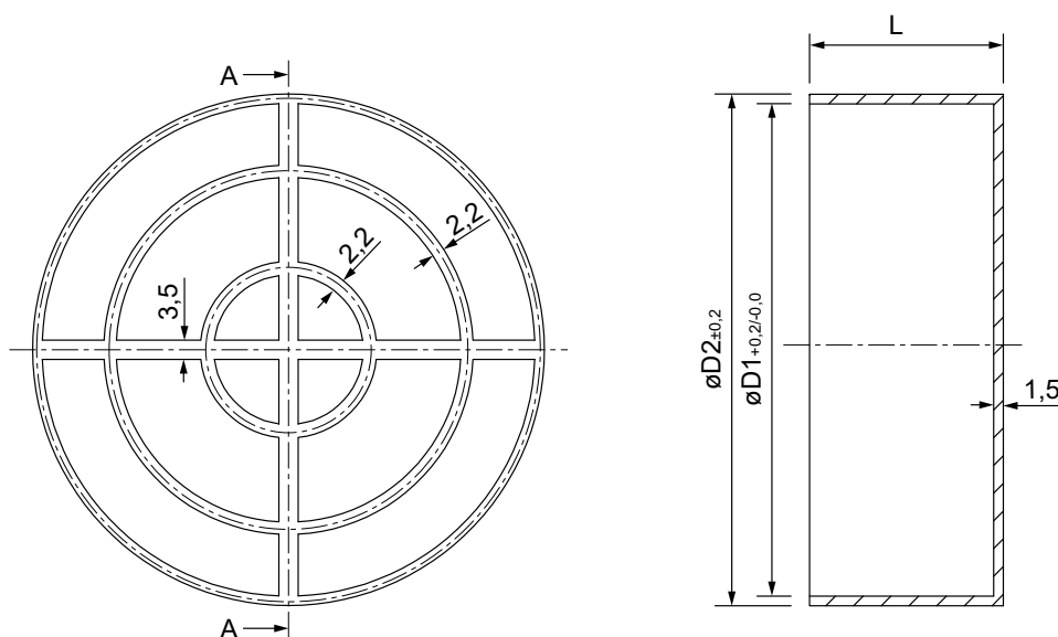
Sec: A-A
